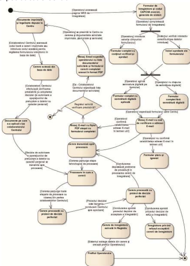
Figura 5. Scenariul expedierii cererii de înregistrare
