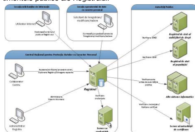
Figura 1. Arhitectura sistemului informațional automatizat
