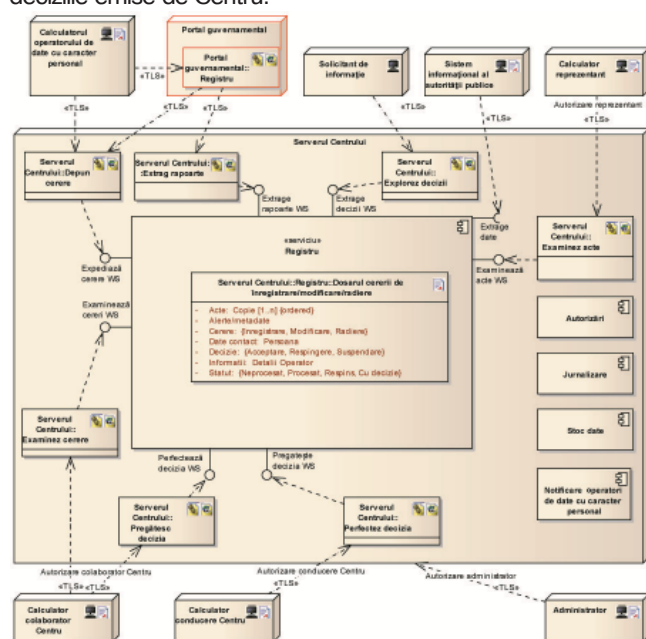
Figura 8. Componentele Sistemului informațional automatizat
